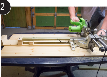
2 Skjære støtteben i riktig lengde
