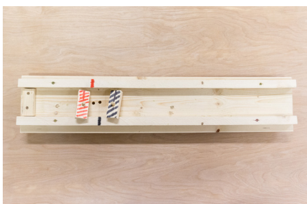
Forboringsjigg skruerull
