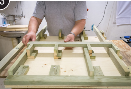
Legg på tverrstøtter
