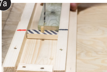
7a Bore skruenhull i alle støtteben, posisjon sort
