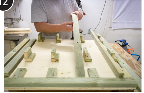
Ben og støtteben i monteringsjigg – side 1
