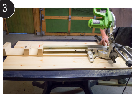
3 Skjær tverrstøtte i riktig lengde
