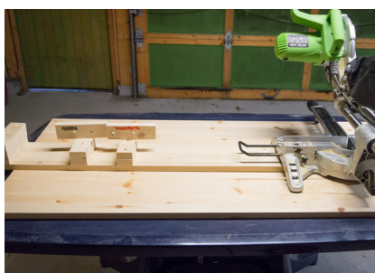
Jigg for kapping av ben, støtteben og tverrstøtte
